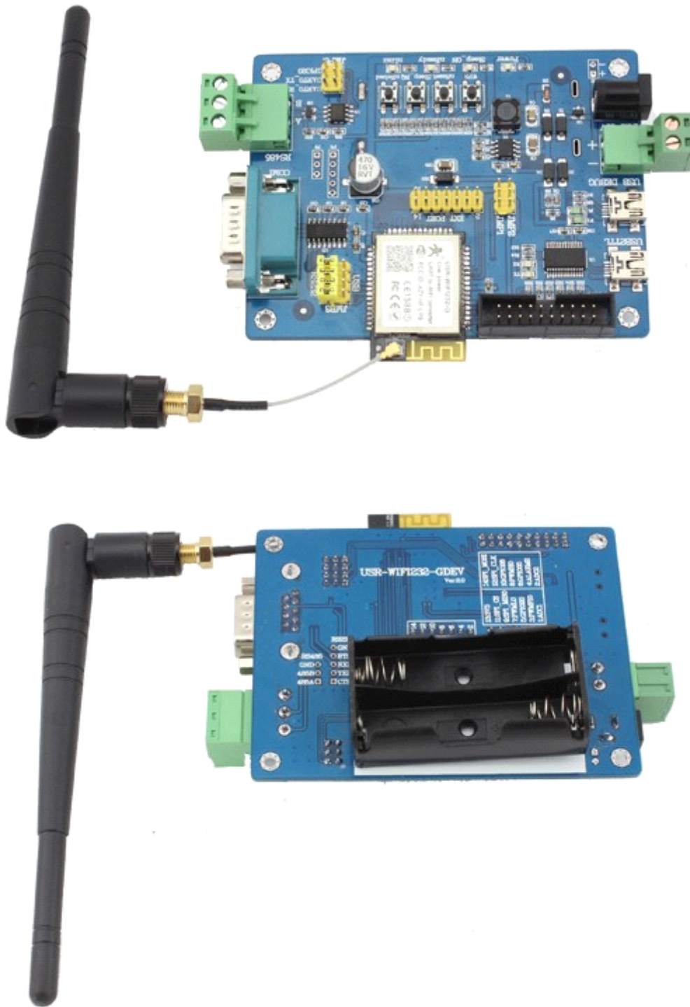
Figure 6. USR-WIFI232-G 开发组件
