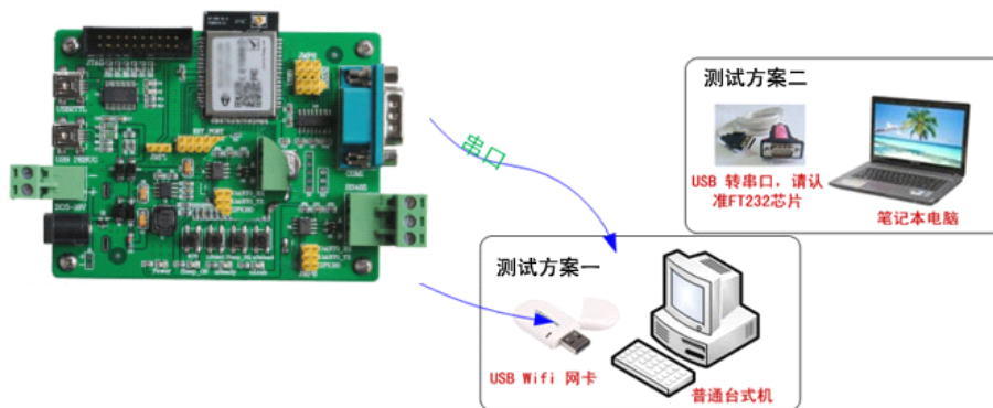
Figure 22. 硬件连接图示
