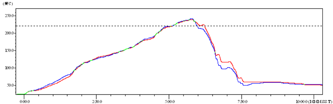
Figure 33. 回流焊焊接温度曲线图
