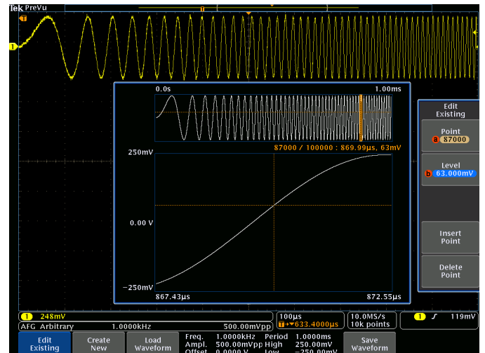
显示点到点编辑的任意波形编辑器。
