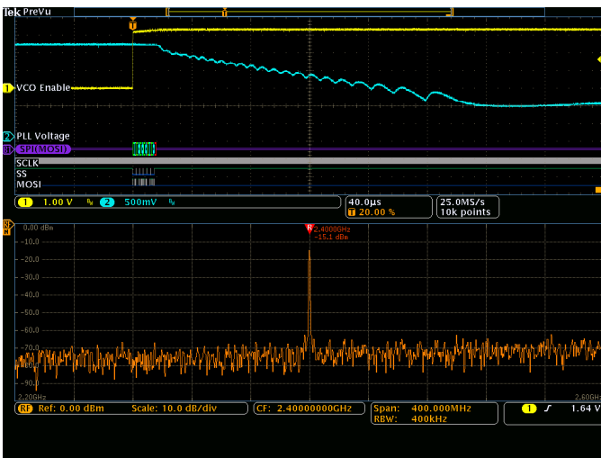
4. 在 VCO 启用大约 320 \mu s 后, PLL 最终稳定在正确的 2.400 GHz 频率上。
