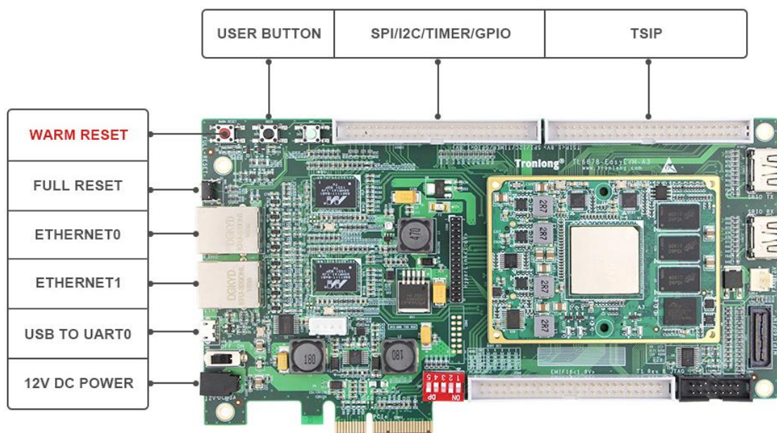
图 8 开发板硬件资源图解 1
