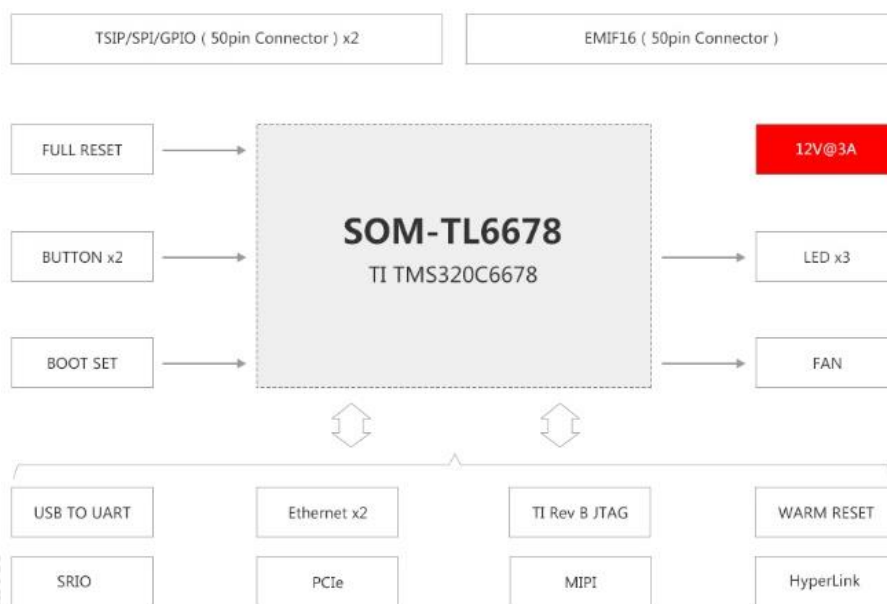
图 7 开发板硬件框图
