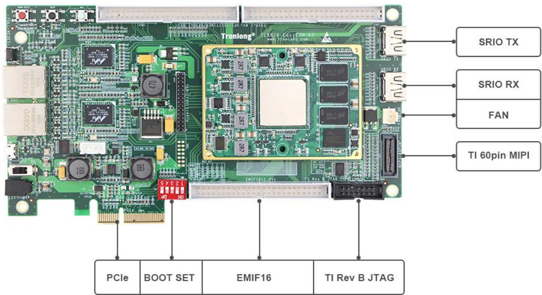
图 9 开发板硬件资源图解 2
