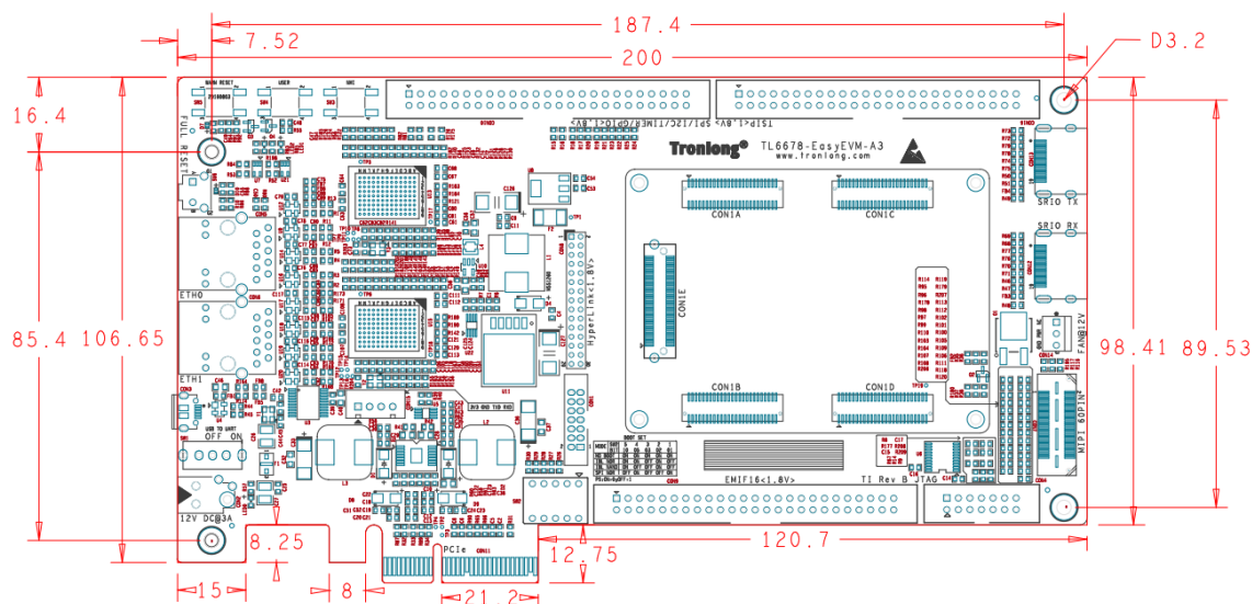
图 11 开发板机械尺寸图
