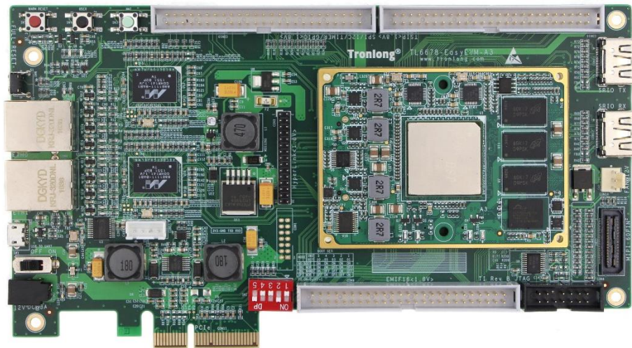
图 1 开发板正面图
