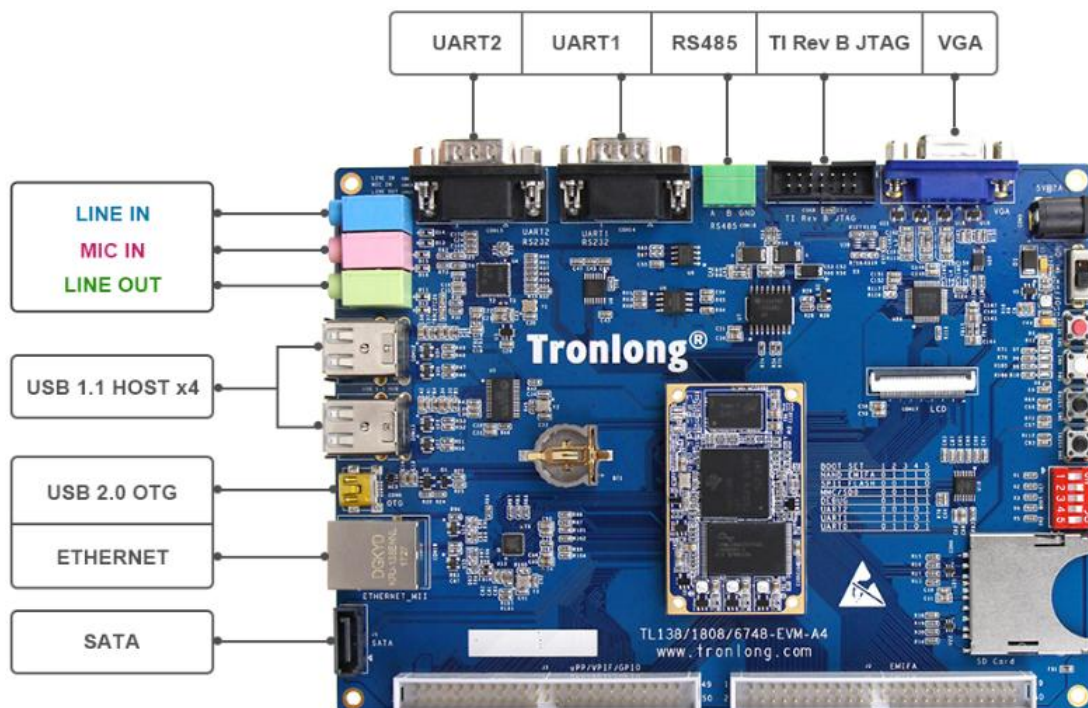
图 9 开发板硬件资源图解 1
