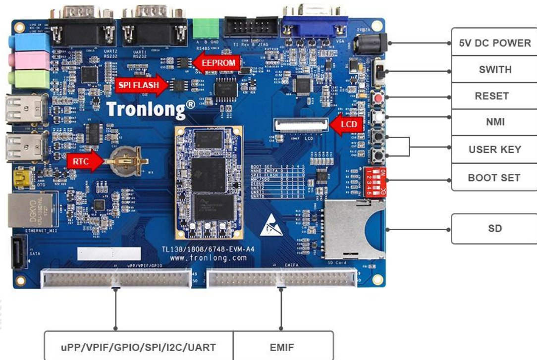
图 10 开发板硬件资源图解 2
