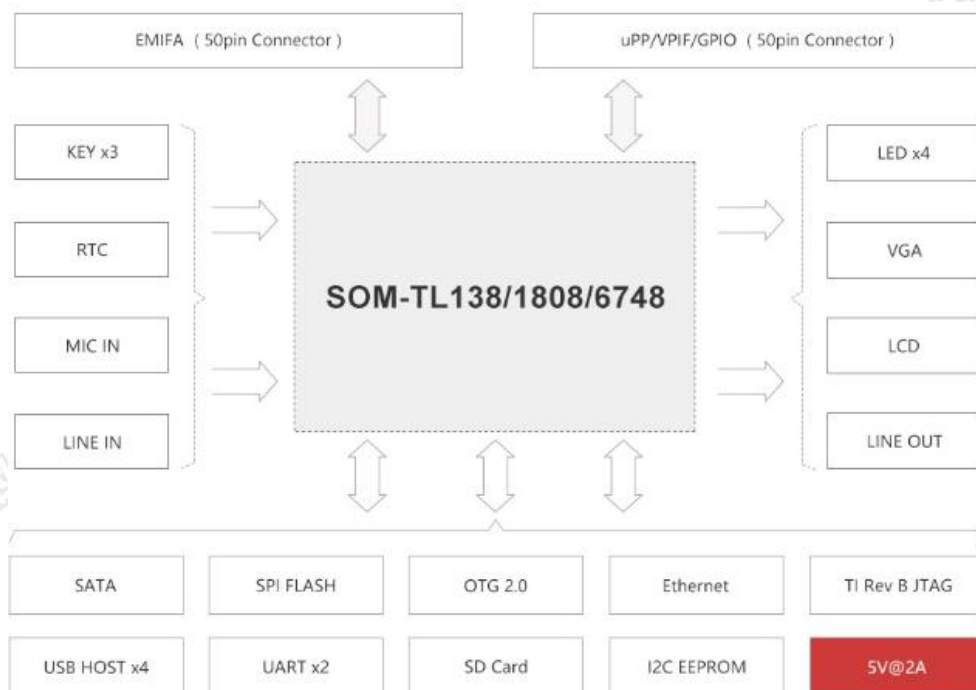
图 8 开发板硬件框图
