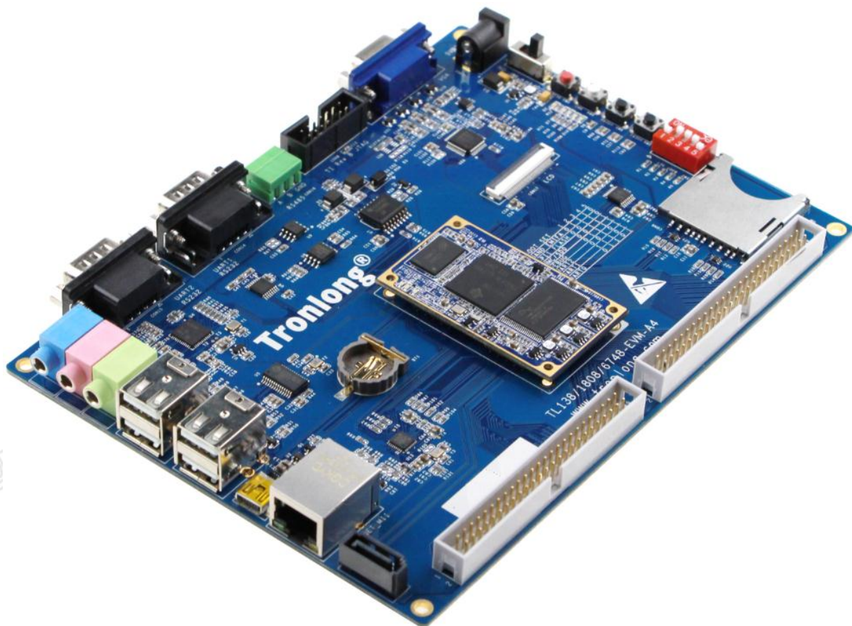
图 3 开发板斜视图
