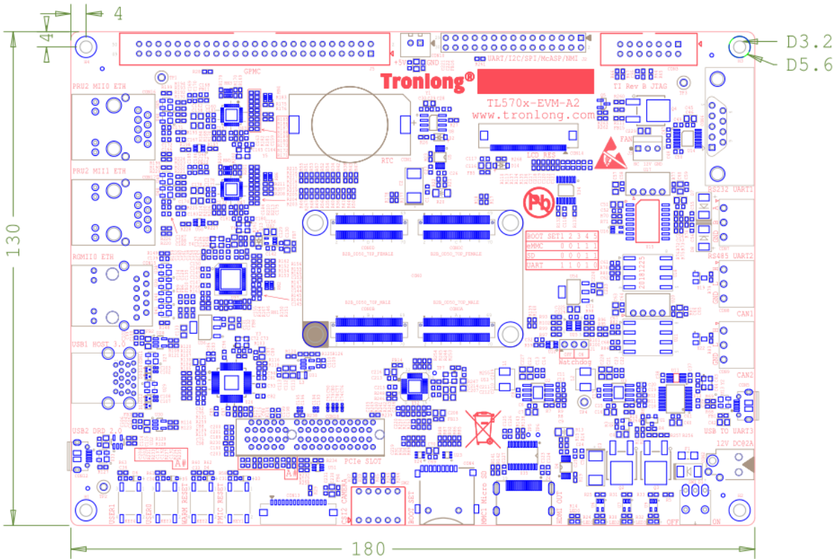
图 12 开发板机械尺寸图
