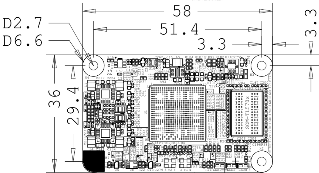
图 11 核心板机械尺寸图
