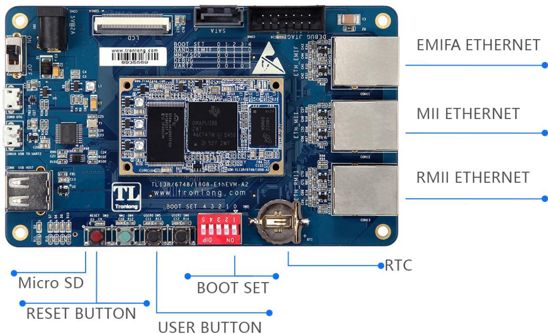
图 11 开发板硬件资源图解 2
