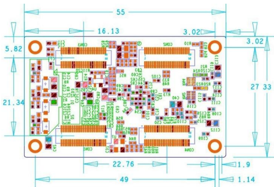
图 12 核心板机械尺寸图
