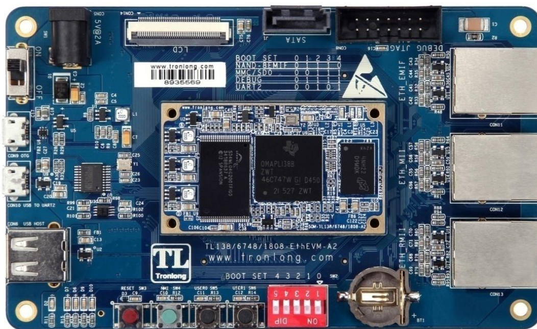
图 1 开发板正面图 1
