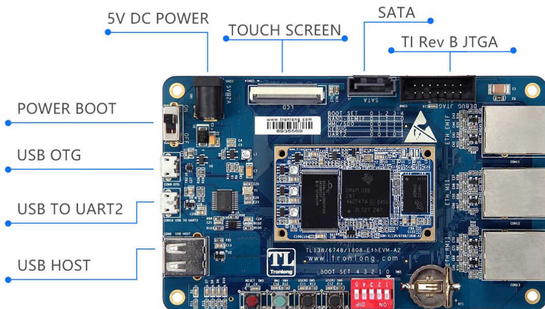
图 10 开发板硬件资源图解 1
