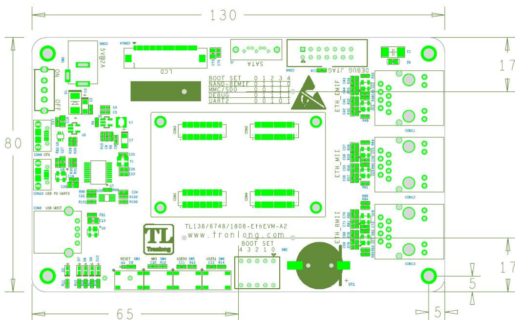
图 13 开发板机械尺寸图
