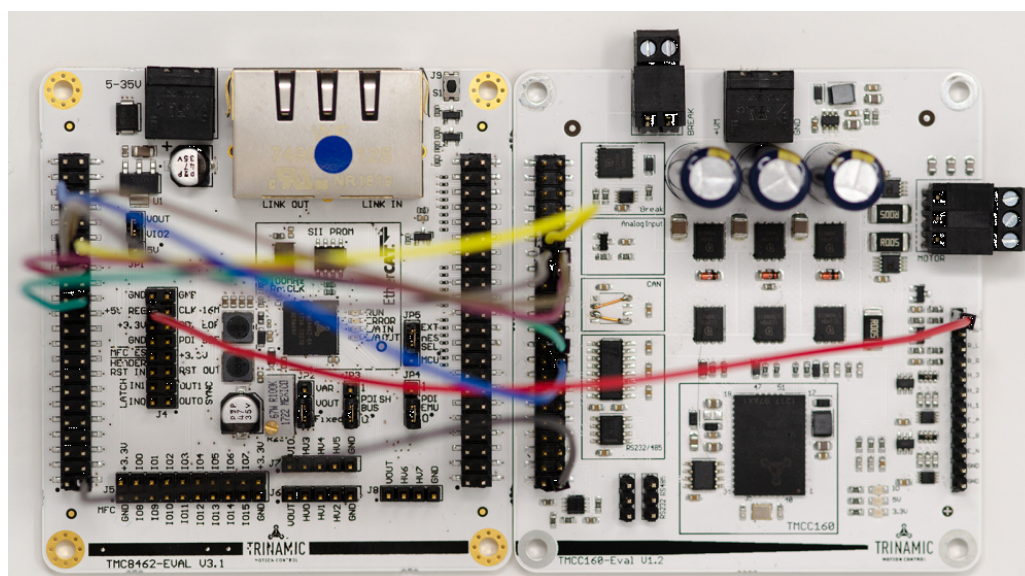
Figure 6: TMCC160-EVAL 开发板 和 TMC8462-EVAL 开发板
