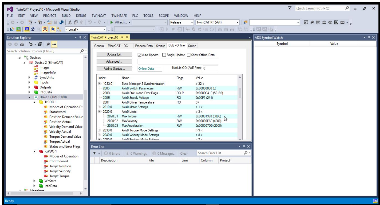
Figure 25: TMCC160-EVAL 在 TwinCAT 显示
