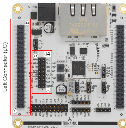
Figure 2: TMCC8462-EVAL 接口
