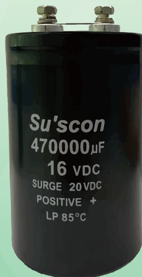
螺丝型
